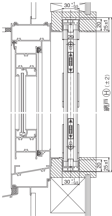
〔縦断面納まり図〕
