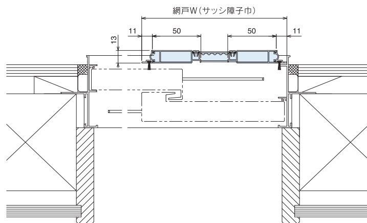
4枚建て召合せ部(テラスタイプ)
