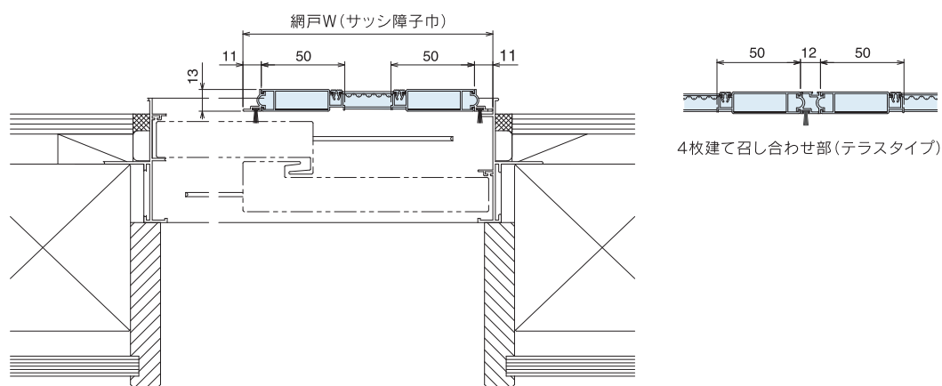
[ 横断面納まり図 ]
