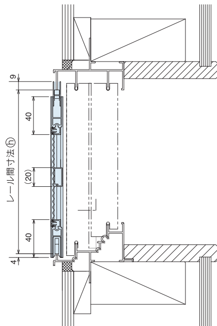
[ 縦断面納まり図 ]
