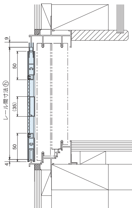
[ 縦断面納まり図 ]
