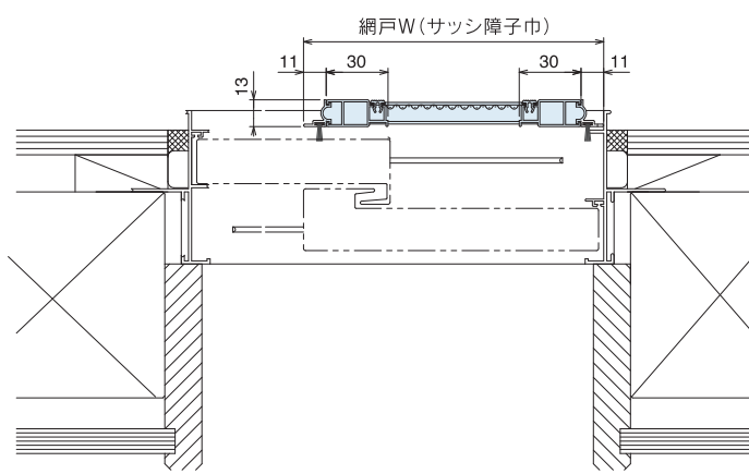
[ 横断面納まり図 ]
