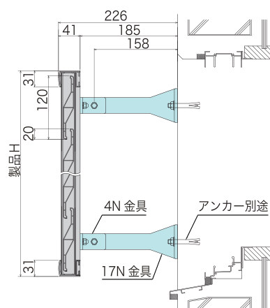
縦断面図
