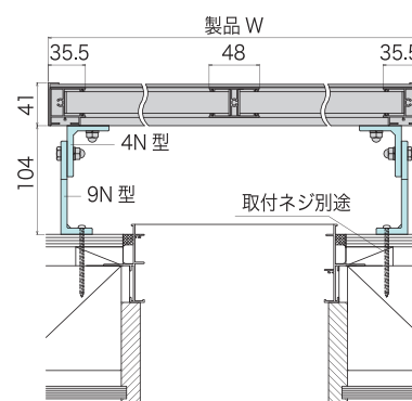
横断面図
