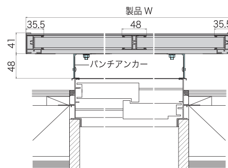
横断面図
