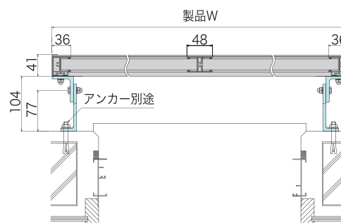
横断面図
