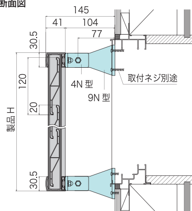
縦断面図
