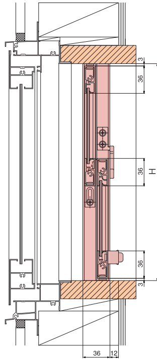
[縦断面納まり図]
