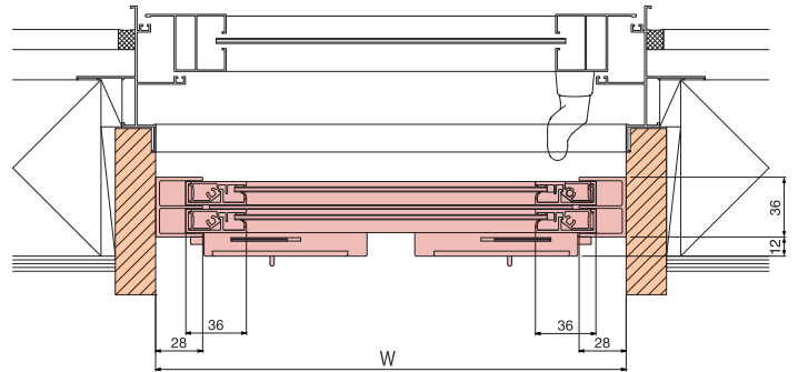
[横断面納まり図]
